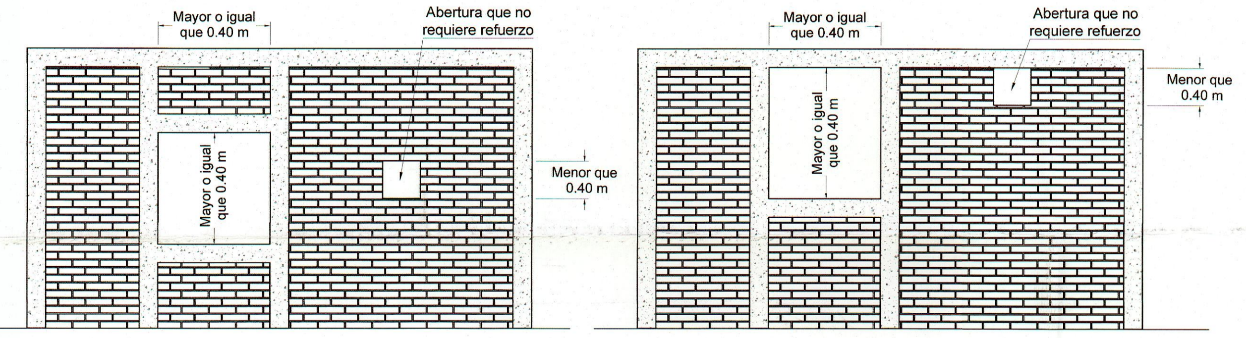
4 REFUERZO EN MUROS CON ABERTURAS ESC-04
