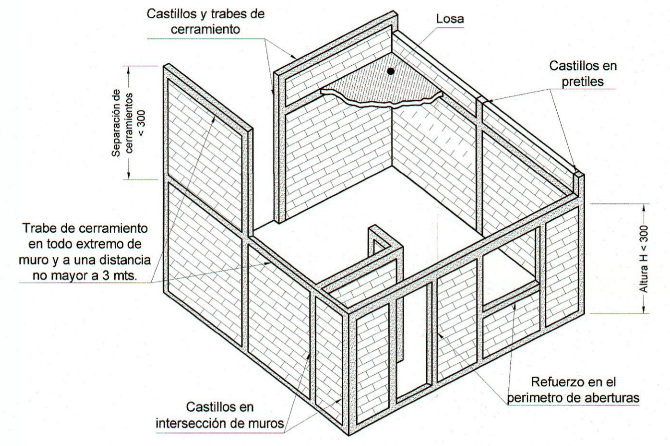
1 MAMPOSTERÍA CONFINADA EN MUROS ESC-04
