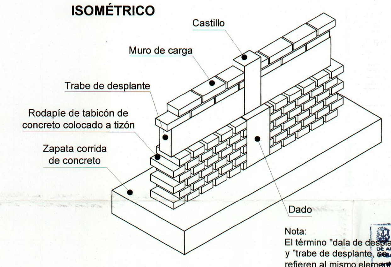
6 SECCIÓN ESTRUCTURAL DE ZAPATA CORRIDA ESC-04
