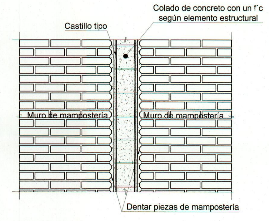
3 COLADO ENTRE MURO DENTADO Y CASTILLO TIPO ESC-04
