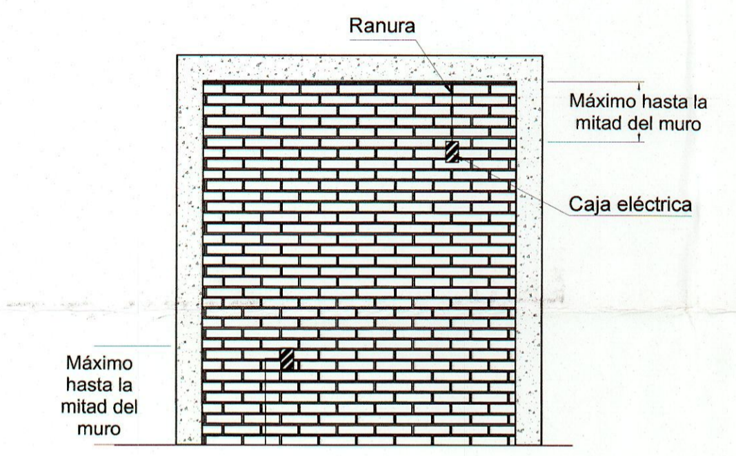
5 RANURADO DE MUROS PARA DUCTOS ELÉCTRICOS ESC-04
